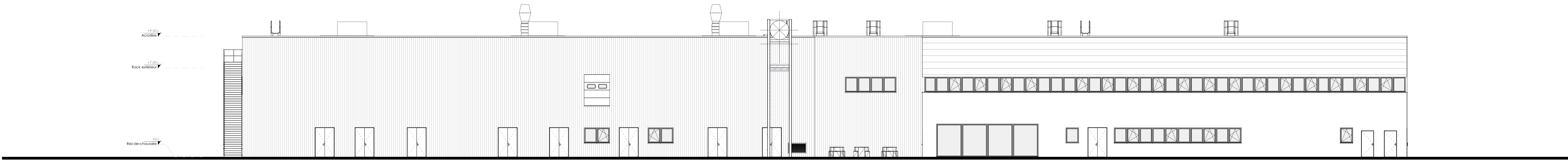
Elévation Est AVP
